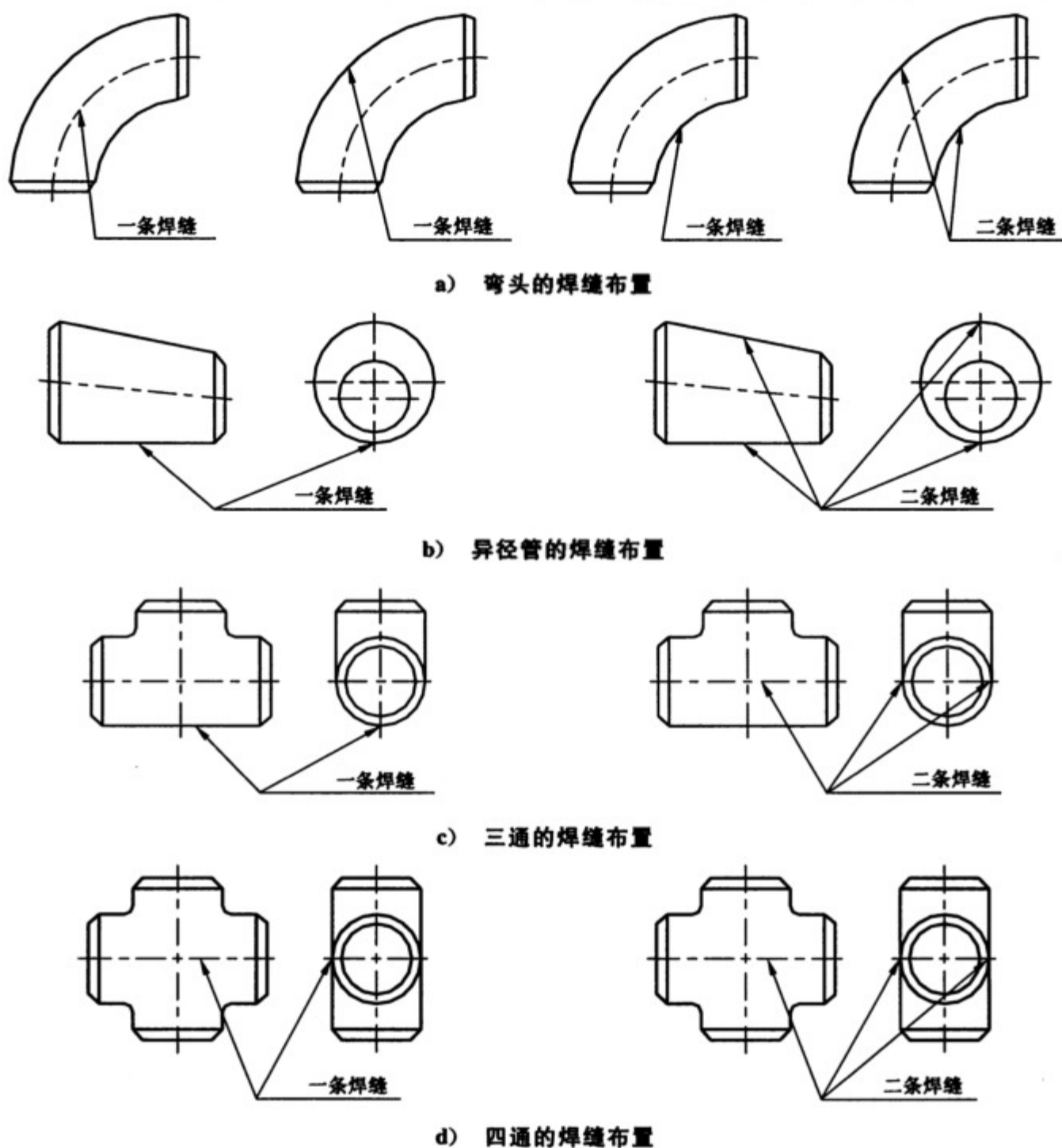
图 1 焊接管件的焊缝布置示意图
